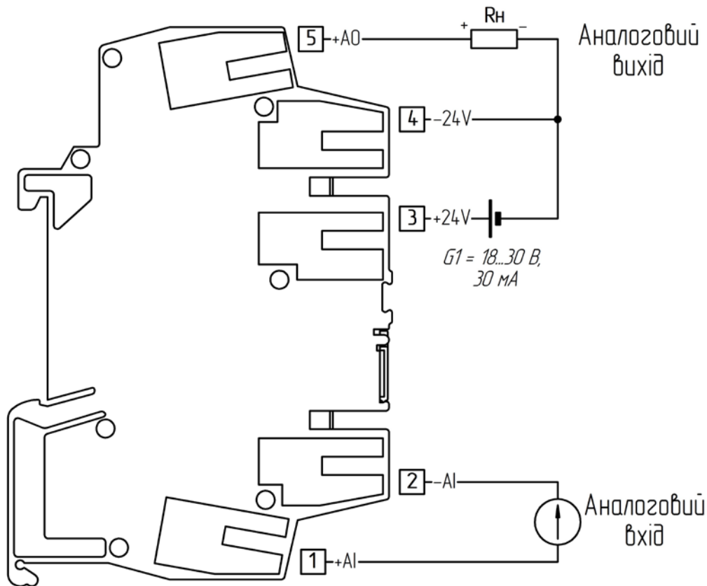
Рисунок 3.4 - Схема зовнішніх з'єднань перетворювача ПНС-651
