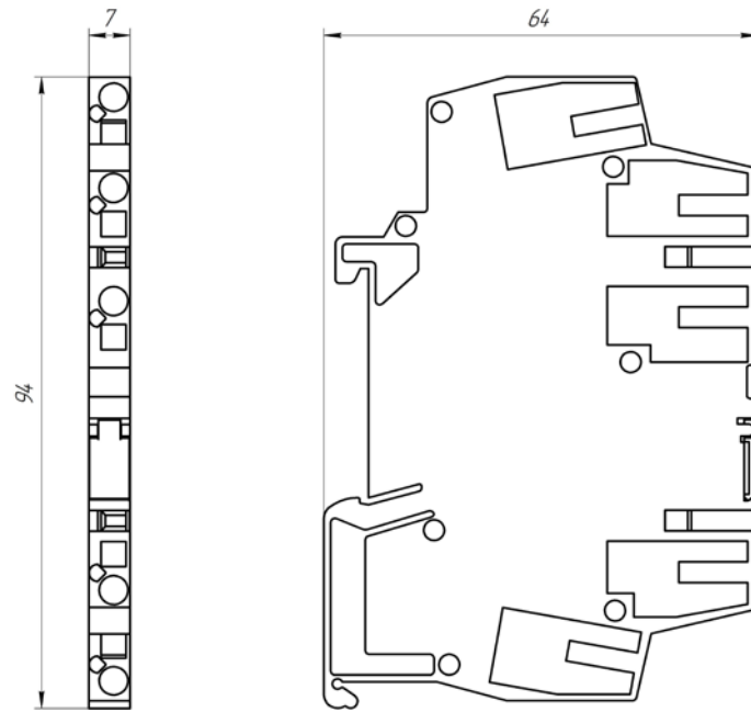
Рисунок 1.1 - Зовнішній вигляд і габаритні розміри перетворювача ПНС-651
