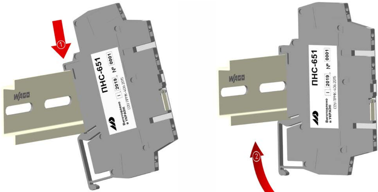
Рисунок 3.2 - Схема кріплення перетворювача ПНС-651 на DIN-рейку
