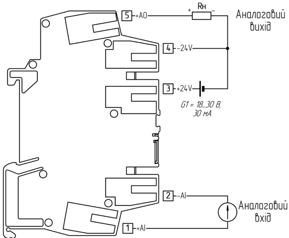
Рисунок 3.4 - Схема зовнішніх з'єднань перетворювача ПНС-650
