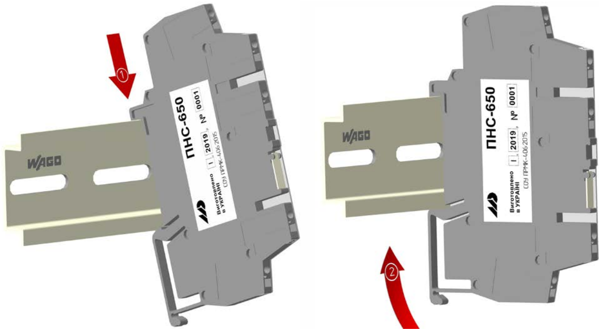
Рисунок 3.2 - Схема кріплення перетворювача ПНС-650 на DIN-рейку
