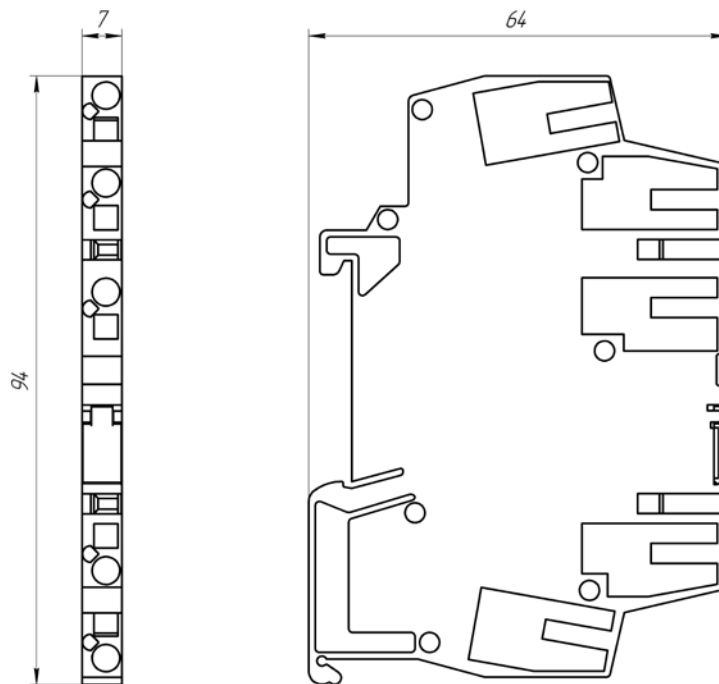
Рисунок 1.1 - Зовнішній вигляд і габаритні розміри перетворювача ПНС-650
