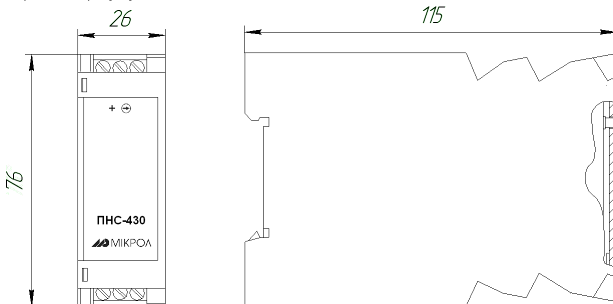
Рисунок 1.1 - Зовнішній вигляд та габаритні розміри ПНС-430
