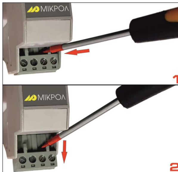
Рисунок 3.3 – Схема виймання роз'єму-кlemi з допомогою плоскої викрутки
