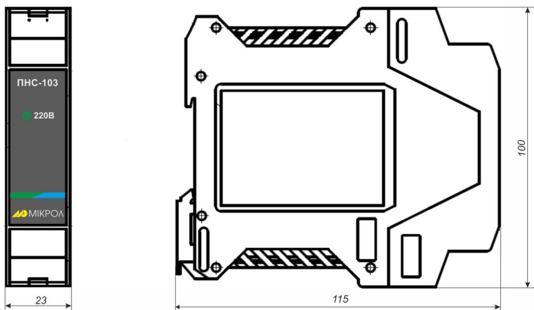
Рисунок 1.1 - Зовнішній вигляд і габаритні розміри БПО-103
