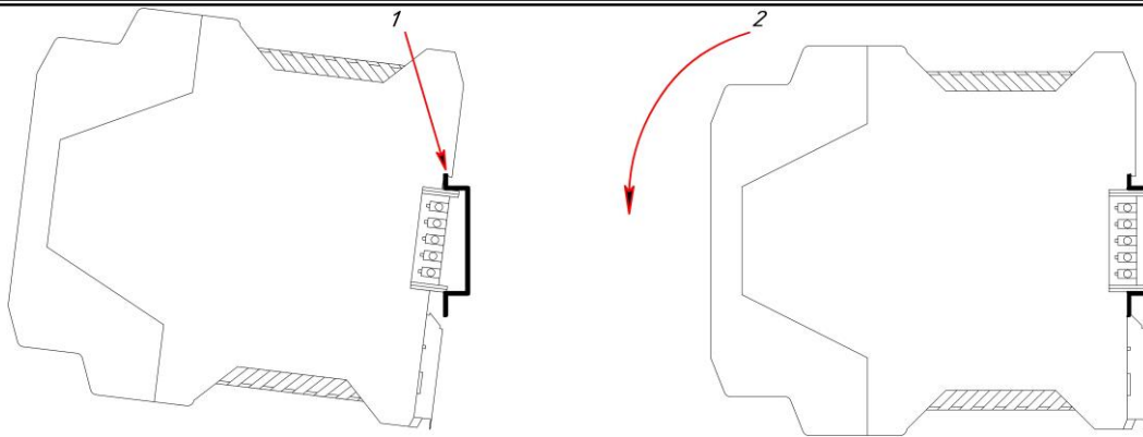
Рисунок 3.2 - Схема кріплення перетворювача ПНС-103 на DIN-рейці
