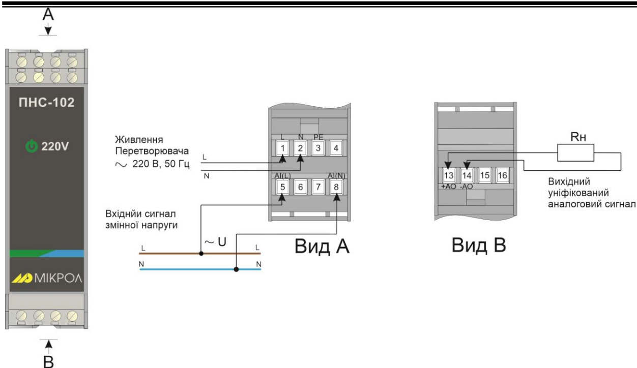
Рисунок 3.4 - Схема електрична підключень перетворювача ПНС-102
