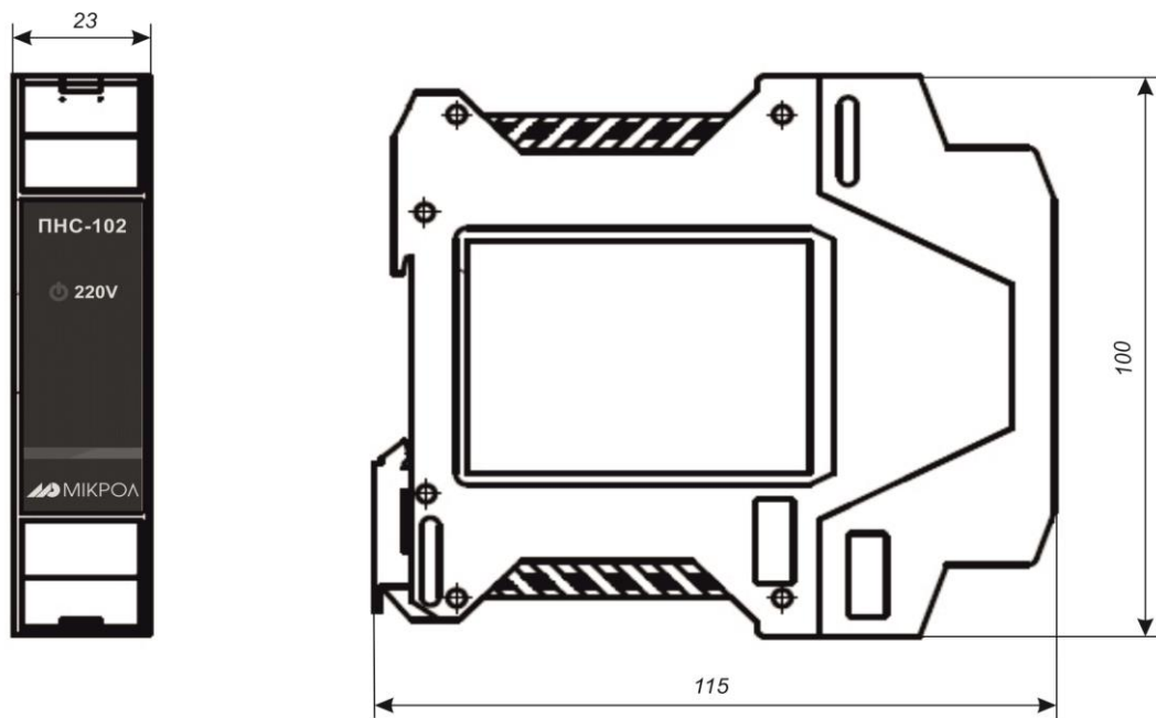
Рисунок 1.1 - Зовнішній вигляд і габаритні розміри БПО-102
