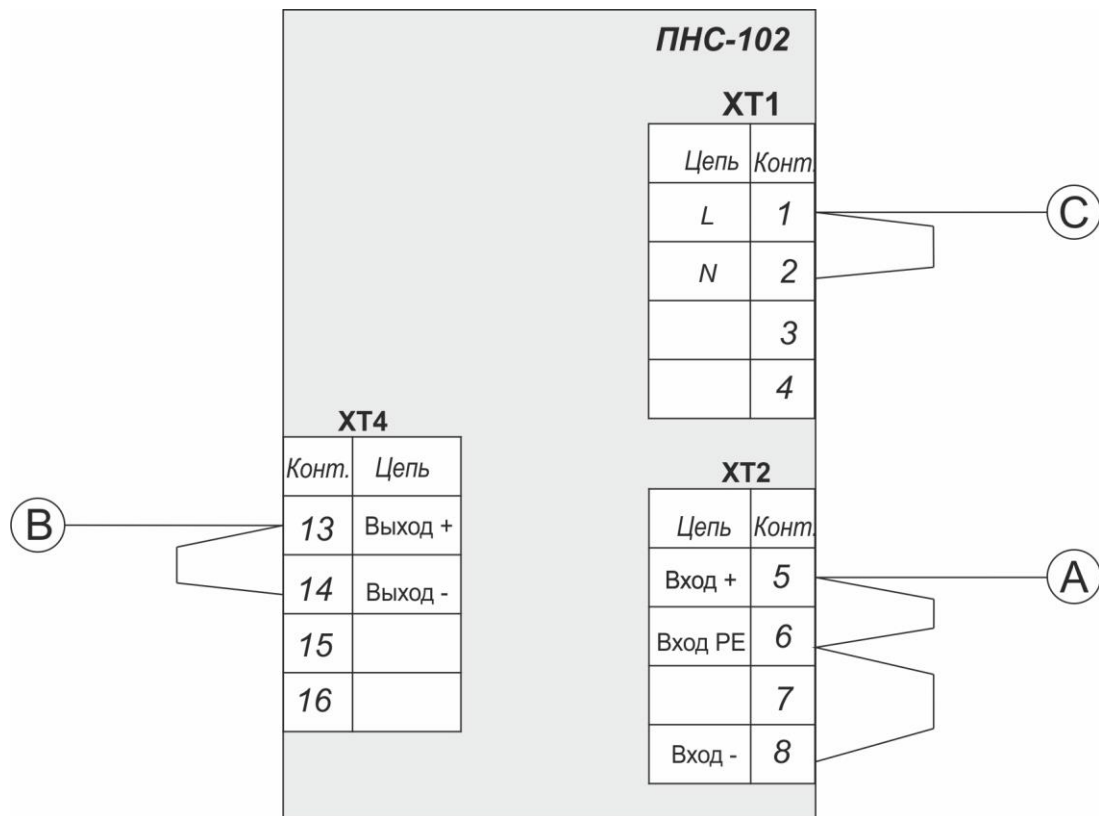
Рисунок Б.1 - Схема перевірки опору ізоляції
