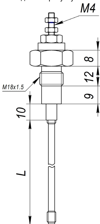
Рисунок 1 – Зовнішній вигляд і габаритні розміри ДК-11
