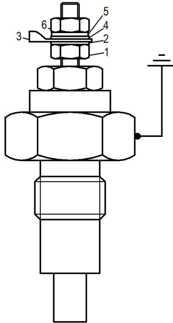
Рисунок 2 - Підключення проводів до полюсів конектора тримача ДК-11
