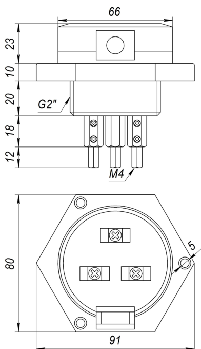
Рисунок 1 — Зовнішній вигляд і габаритні розміри ДК-3
