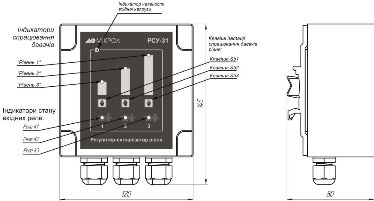
Рисунок 1.4 — вигляд і габаритні розміри PCY-31
