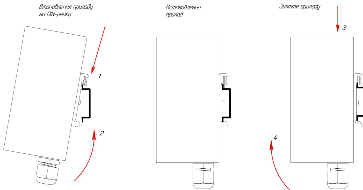
Рисунок 4.1 — Схема встановлення і зняття блоку РСУ-31
