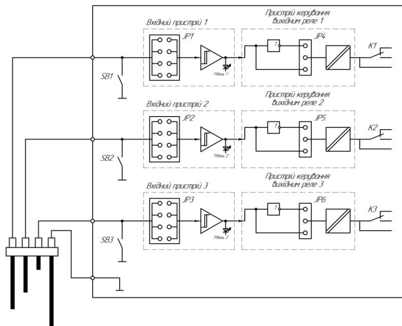
Рисунок 2.2 - Функціональна схема блоку РСУ-31
