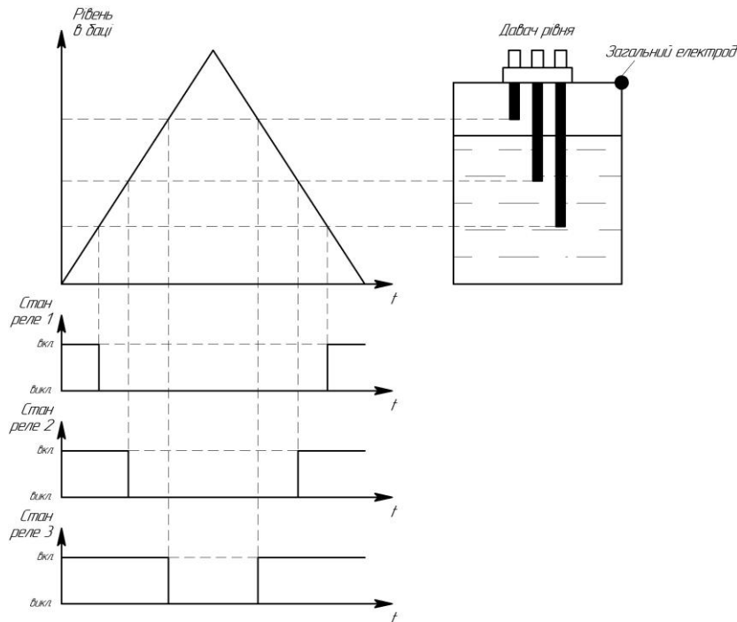
Рисунок 2.3 - Діаграма роботи блоку РСУ-31
