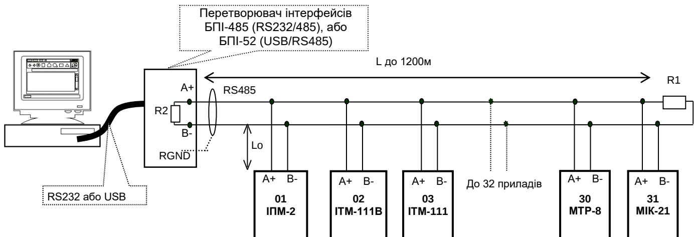
Рисунок Б.3 - Організація інтерфейсного зв'язку між комп'ютером та вольтметрами або контролерами
