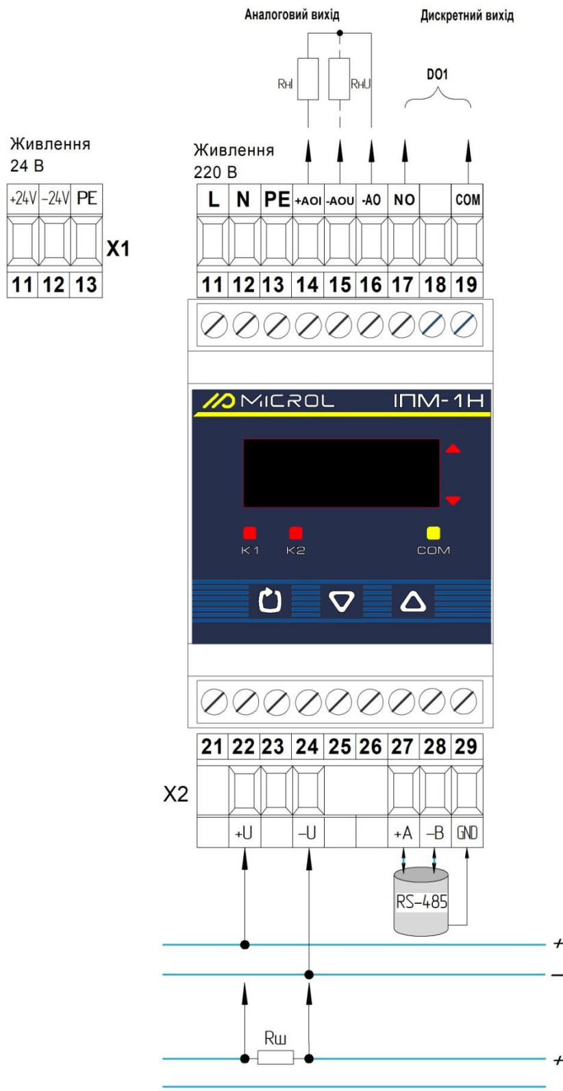
Рисунок Б.1 Підключення зовнішніх ланцюгів до вольтметра ІПМ-1Н:
