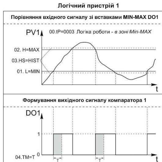
Рисунок 3.7 – Функціональна схема принципу роботи DO як компаратора
