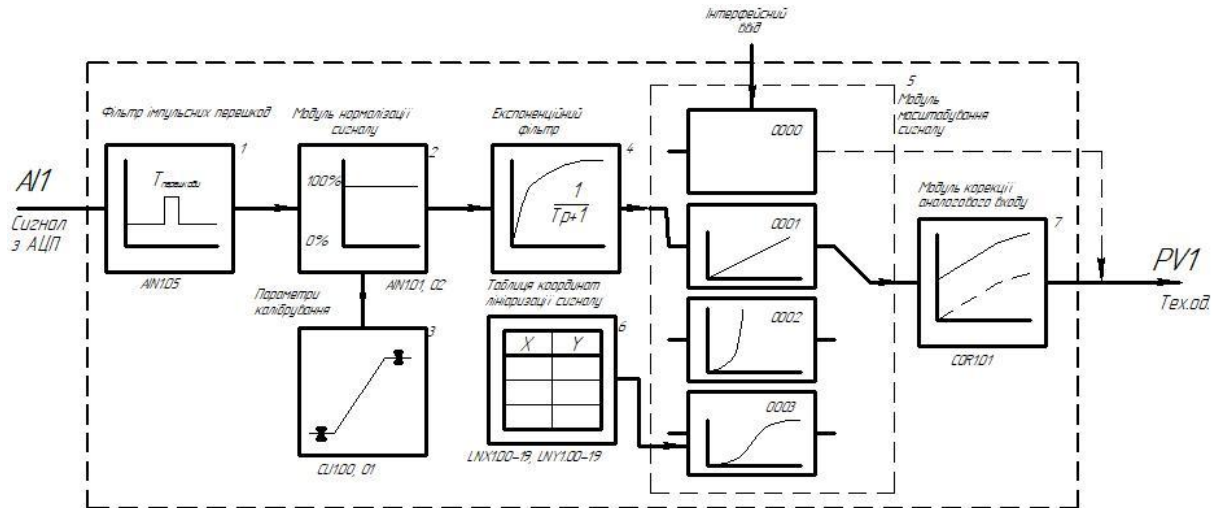
Рисунок 3.4 – Блок-схема обробки аналогового входу
