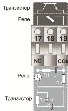
Рисунок Б.2 - Підключення дискретних виходів до вольтметра ІПМ-1Н:
