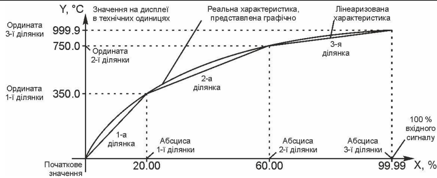
Рисунок 3.5 – Графік лінеаризованого сигналу
