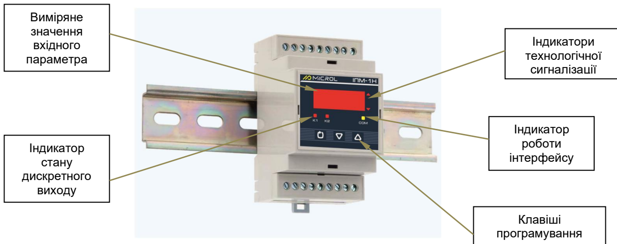
Рисунок 3.1 – Зовнішній вигляд вольтметра ІПМ-1Н
