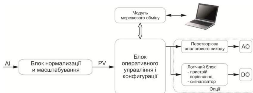
Рисунок 3.3 – Функціональна схема вольтметра ІПМ-1Н
