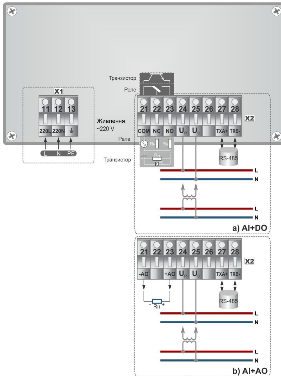
Рисунок Б.1 - Підключення зовнішніх ланцюгів до вольтметра ІПМ-2: а) підключення за умови замовлення опції дискретного виходу; б) підключення за умови замовлення опції аналогового виходу.
