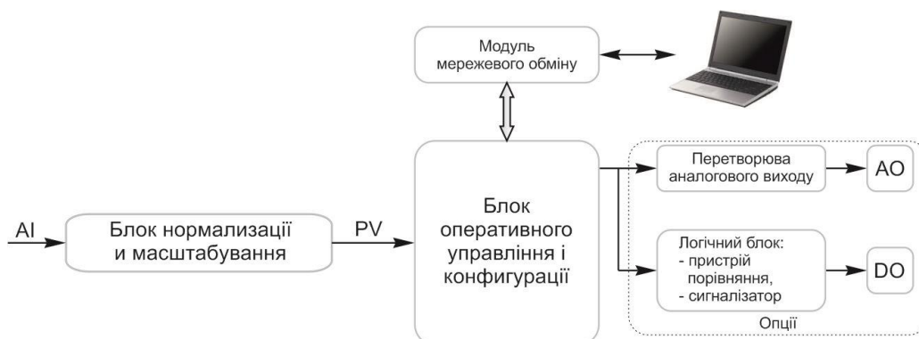
Рисунок 3.3 – Функціональна схема вольтметра ІПМ-2
