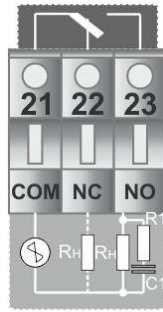
Рисунок Б.2 – Схема підключення індуктивного навантаження до механічного реле
