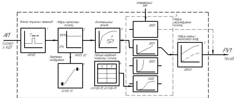
Рисунок 3.4 – Блок-схема обробки аналогового входу
