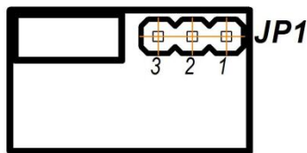
Рисунок 5.1 – Положення перемичок на модулі аналогового виходу
