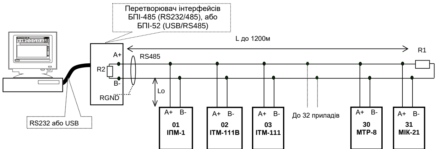
Рисунок Б.3 - Організація інтерфейсного зв'язку між комп'ютером та вольтметрами або контролерами
