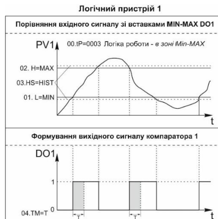
Рисунок 3.7 – Функціональна схема принципу роботи DO як компаратора
