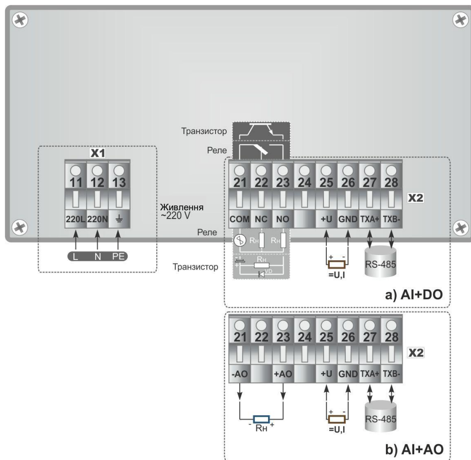
Рисунок Б.1 -Підключення зовнішніх панцюгів до вольтметра ІПМ-1: а) підключення за умови замовлення опції дискретного виходу; б) підключення за умови замовлення опції аналогового виходу.
