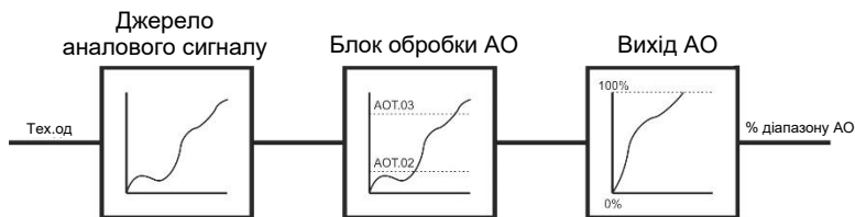
Рисунок 3.6 – Робота блоку аналогового виведення у режимі лінійного перетворення
