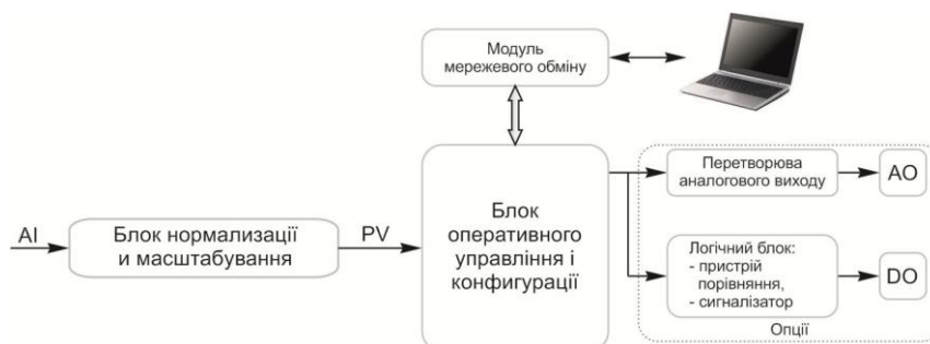
Рисунок 3.3 – Функціональна схема вольтметра ІПМ-1
