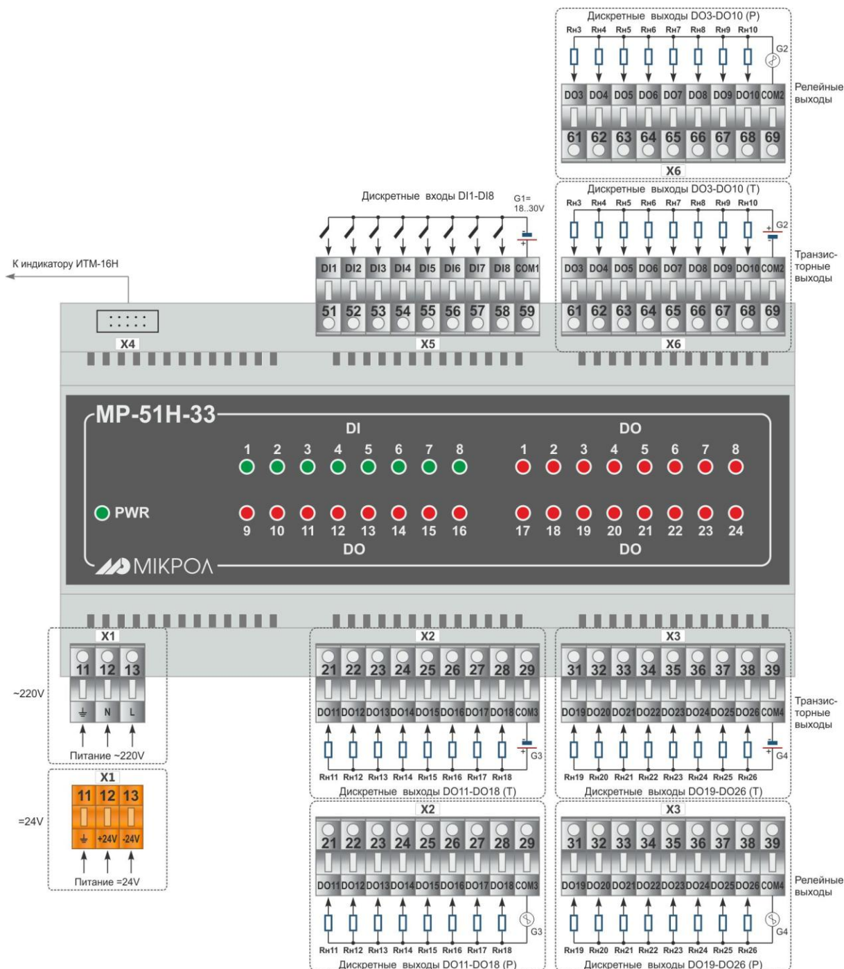
Рисунок Б.13 - Схема зовнішніх з'єднань модуля розширення MP-51H-33
