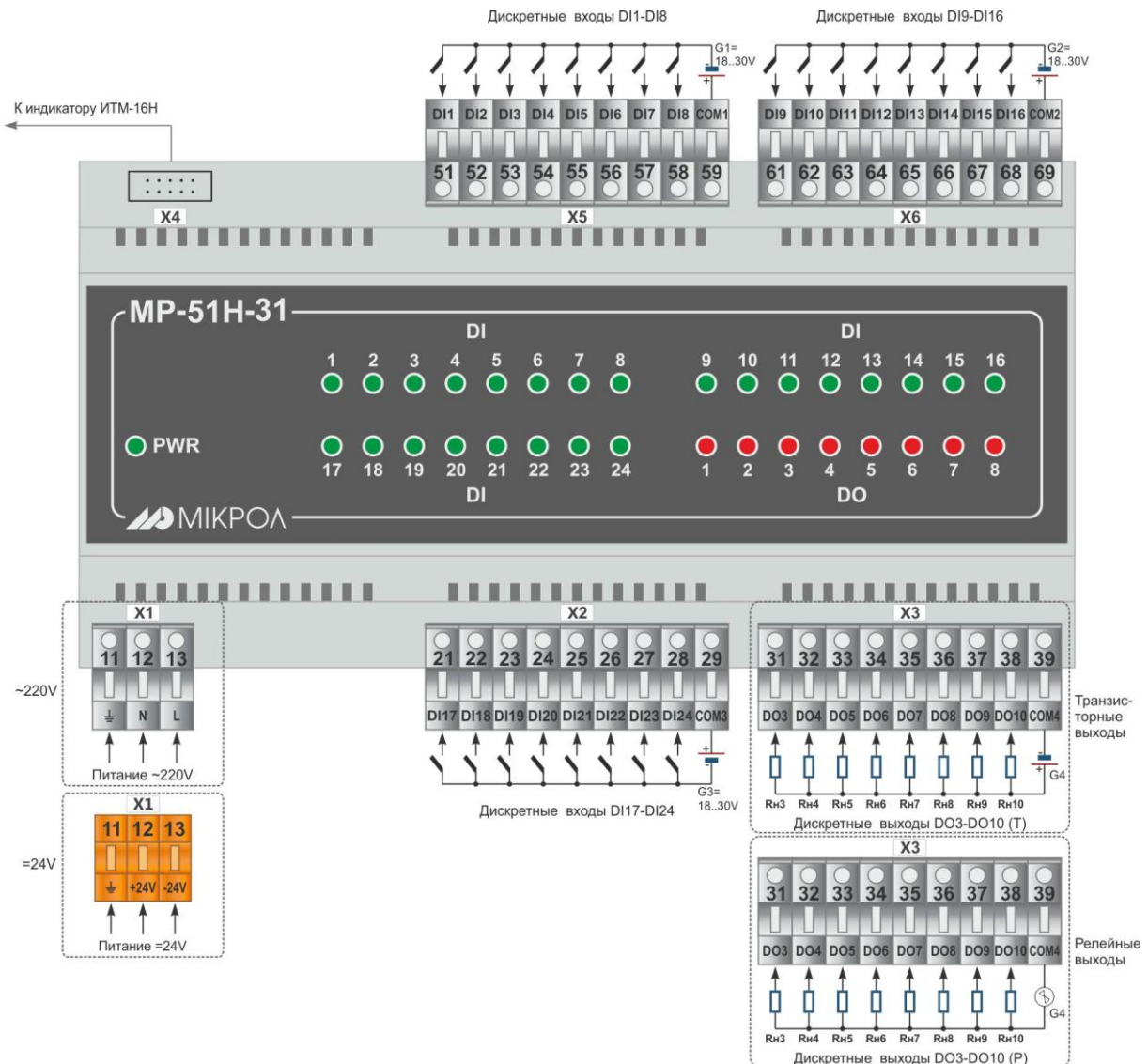
Рисунок Б.11 - Схема зовнішніх з'єднань модуля розширення MP-51H-31
