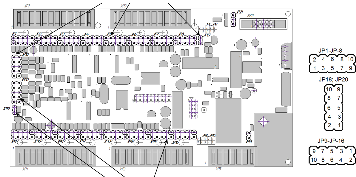
Перемички 9-16 аналогових входів
