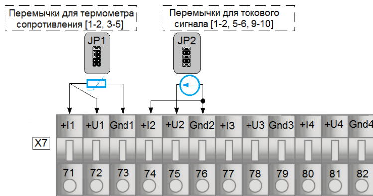
Рисунок 4.4 - Підключення давача постійного струму (при одночасному підключенні термометрів опору до обраної групи аналогових входів)
