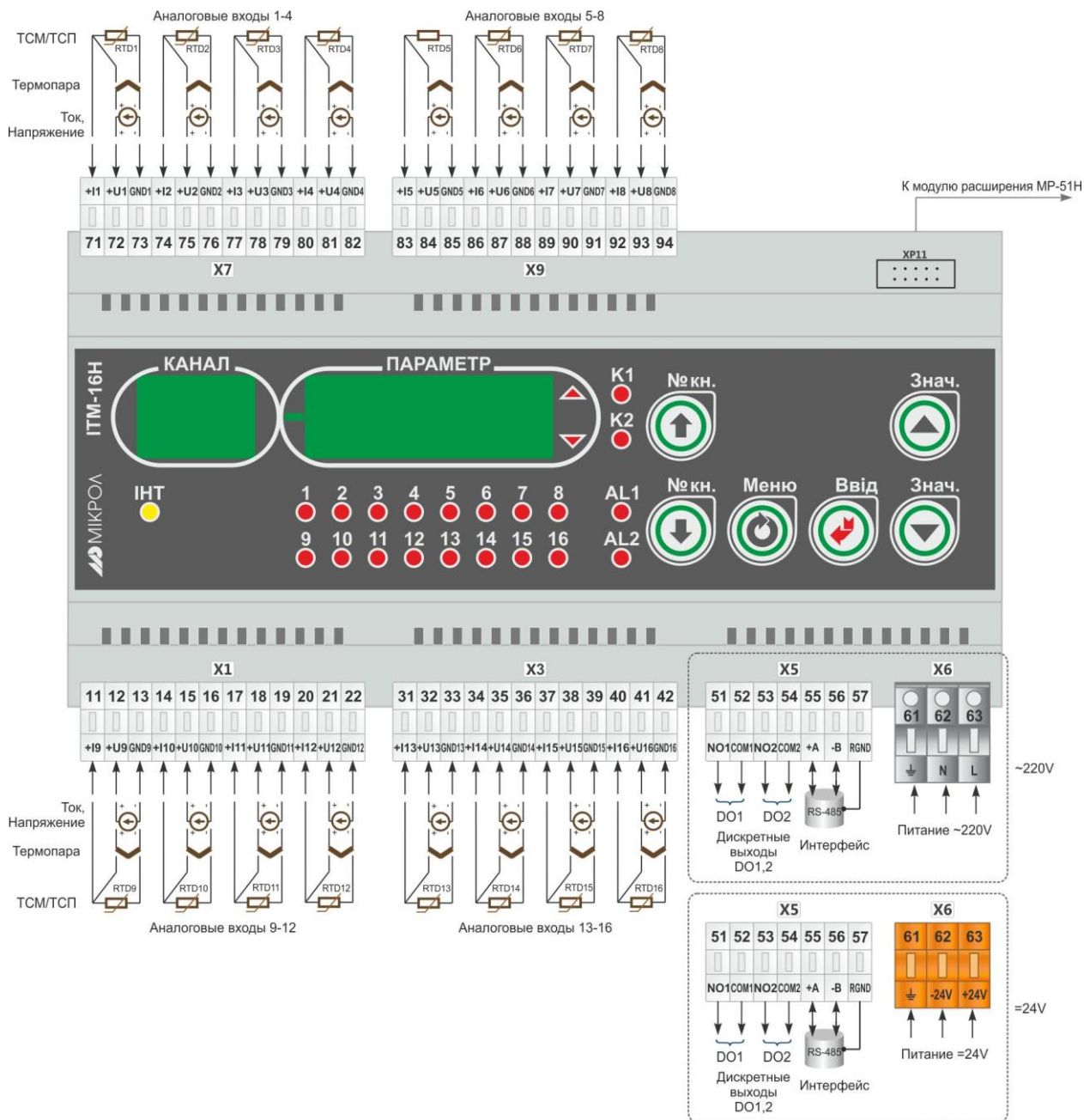
Рисунок Б.1 -Підключення зовнішніх ланцюгів до індикатора ІТМ-16Н
