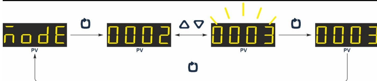
Рисунок 4.4 – Фіксація зміни параметру індикатора ITM-311(B)
