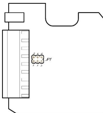
Рисунок 4.6 - Положення перемичок на платі приладу
