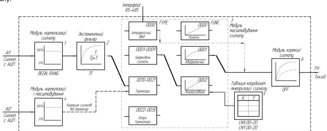
Рисунок 3.3 - Функціональна схема блоку перетворення вхідного сигналу
