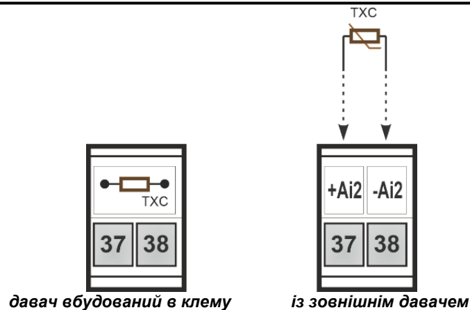
Рисунок Б.3.4 – Підключення давача термокомпенсації в залежності від замовлення версії приладу
