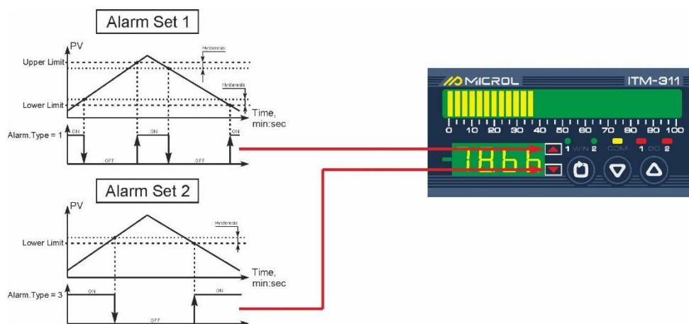
Рисунок 3.4 – Принцип роботи сигналізації
