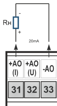
Рисунок Б.4.3 – Схема підключення виходу постійного струму
