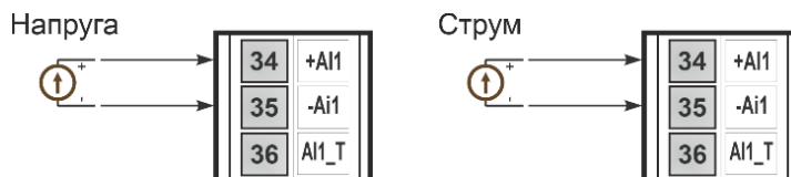
Рисунок Б.3.5 - Схема підключення уніфікованих сигналів активного типу
