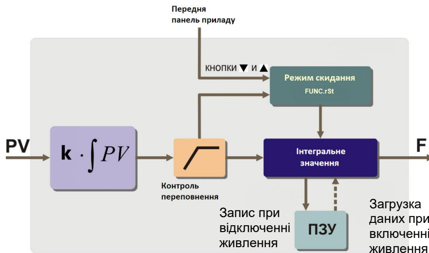
Рисунок 3.6 - Блок-схема функції інтегрування
