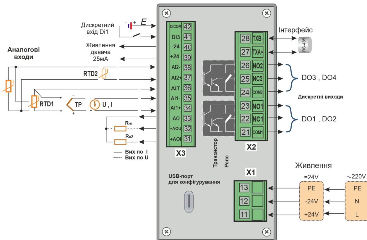
Рисунок Б.2 - Схема зовнішніх з'єднань індикатора ІТМ-311В
