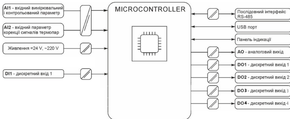
Рисунок 3.2 - Структурна схема індикатора ITM-311(B)
