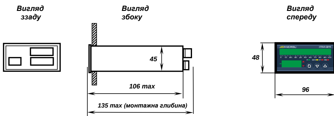
Рисунок А.1 – Зовнішній вигляд індикатора ІТМ-311(В) та розміри цифрових індикаторів
