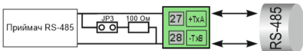
Рисунок Б.5.2 - Організація внутрішнього з'єднання інтерфейсу RS-485
