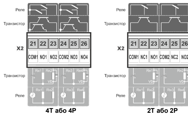
Рисунок Б.4.1 - Підключення дискретних навантажень до індикатора ІТМ-311(В)
