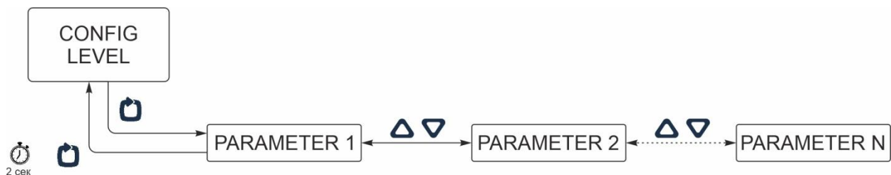
Рисунок 4.3 – Перехід між конфігураційними параметрами індикатора ITM-311(B)
