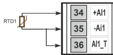
Рисунок Б.3.2 – Двох провідна схема підключення термоопорів
