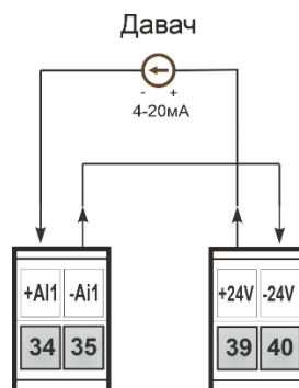
Рисунок Б.3.6 - Схема підключення уніфікованих сигналів пасивного типу при використанні внутрішнього блоку живлення
