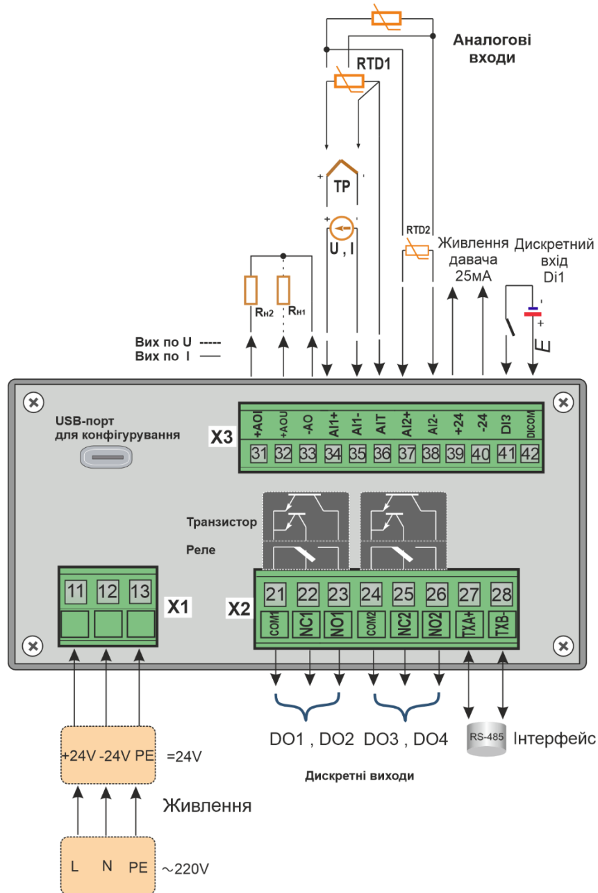
Рисунок Б.1 - Схема зовнішніх з'єднань індикатора ІТМ-311
