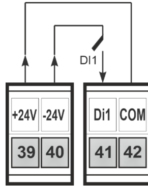
Рисунок Б.3.7 - Схема підключення дискретних вхідних сигналів
