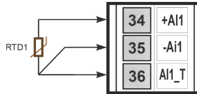
Рисунок Б.3.1 – Трьох провідна схема підключення термоопорів
