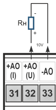
Рисунок Б.4.4 – Схема підключення виходу постійної напруги
