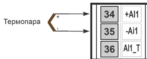
Рисунок Б.3.3 – Схема підключення термопар
