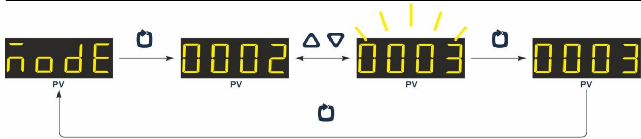
Рисунок 4.4 – Фіксація зміни параметру індикатора ITM-310(ITM-310A)
