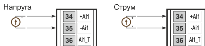
Рисунок Б.2.5 - Схема підключення уніфікованих сигналів активного типу
