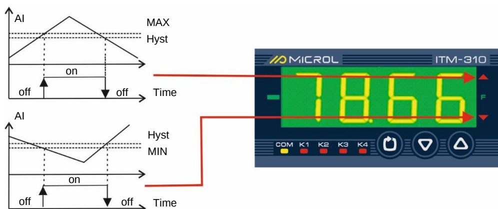
Рисунок 3.5 – Принцип роботи сигналізації
