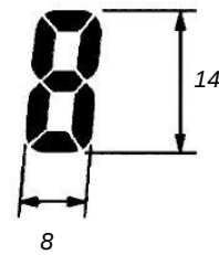
Рисунок А.2 – Зовнішній вигляд індикатора ITM-310A та розміри цифрових індикаторів (тип індикаторів - 1)
