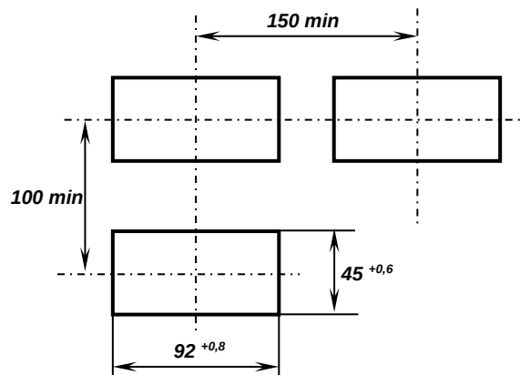
Рисунок А.4 – Розмітка отворів на щиті для встановлення індикатора
