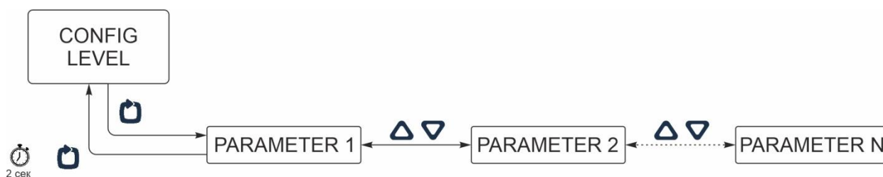
Рисунок 4.3 – Перехід між конфігураційними параметрами індикатора ITM-310(ITM-310A)
