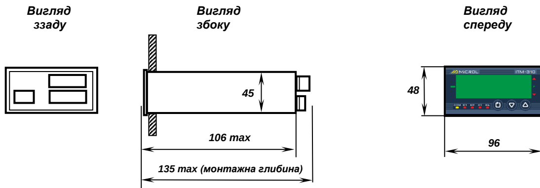
Рисунок А.3 – Габаритні розміри індикатора
