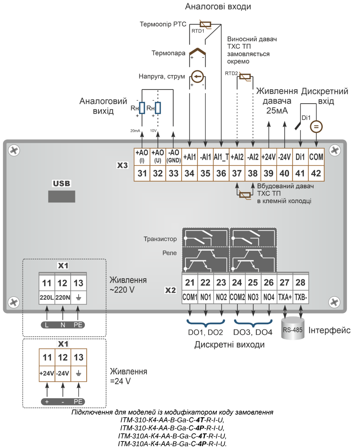
Рисунок Б.2 - Схема зовнішніх з'єднань індикатора ITM-310(ITM-310A)
