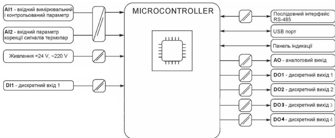
Рисунок 3.3 - Структурна схема індикатора ITM-310(ITM-310A)
