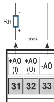
Рисунок Б.3.5 – Схема підключення виходу постійного струму
