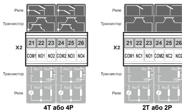
Рисунок Б.3.1 - Підключення дискретних навантажень до індикатора ITM-310(ITM-310A)
