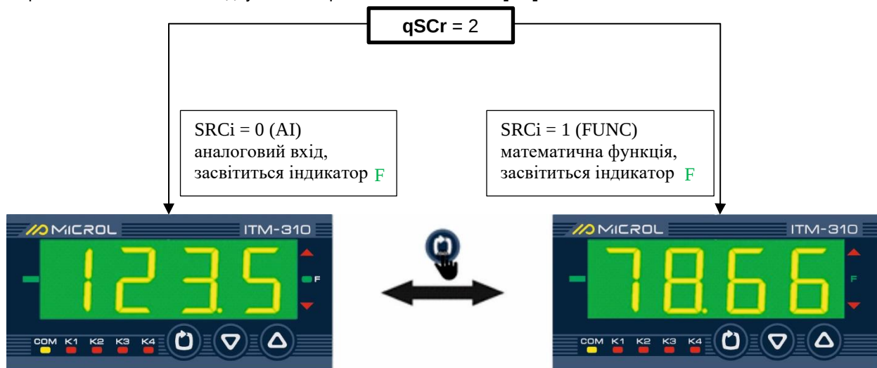
Рисунок 3.7 - Блок-схема роботи вікон відображення
