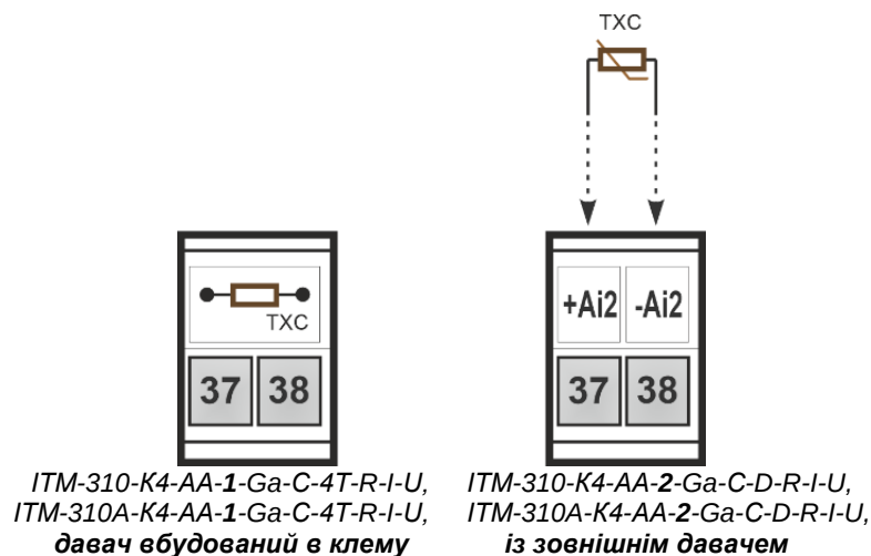
Рисунок Б.2.4 – Підключення датчика термокомпенсації в залежності від замовлення версії приладу
