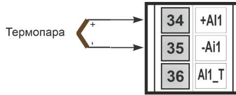
Рисунок Б.2.3 – Схема підключення термопар
