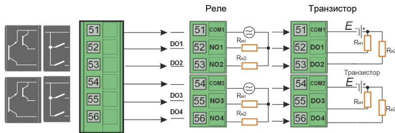
Рисунок Б.3.1 - Підключення дискретних навантажень до індикатора ІТМ-320 (ІТМ-320А)
