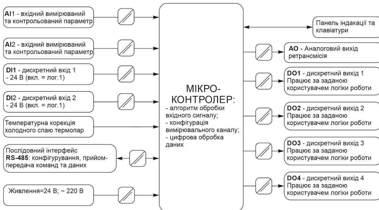
Рисунок 3.2 – Структурна схема індикатора ITM-120-K6
