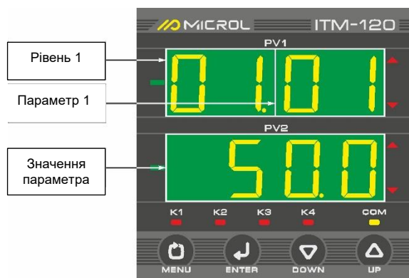
Рисунок 4.3 – Індикація значення параметрів конфігурації та їх номерів
