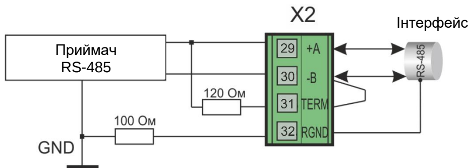
Рисунок Б.7 - Рекомендована схема підключення інтерфейсу RS-485
