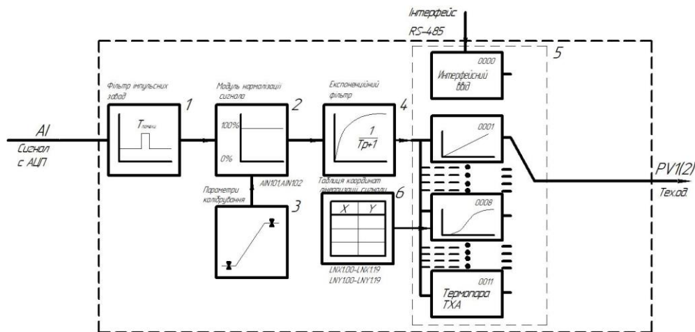
Рисунок 3.4 – Блок-схема обробки аналогового входу
