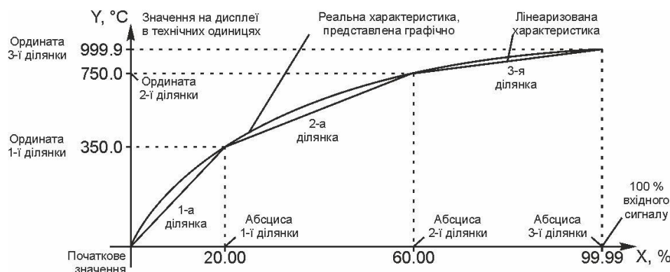
Рисунок 3.5 – Графічне уявлення кривої лінеаризації
