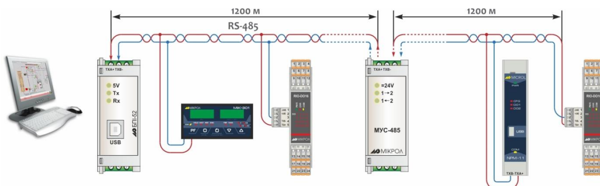
Рисунок Б.6 - Організація інтерфейсного зв'язку між комп'ютером та приладами
