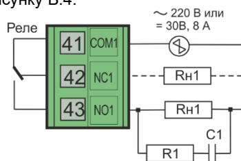
Рисунок Б.4 – Схема підключення індуктивного навантаження для механічного реле
