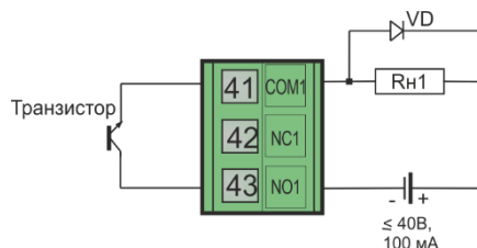
Рисунок Б.3 – Схема підключення індуктивного навантаження для транзисторного виходу
