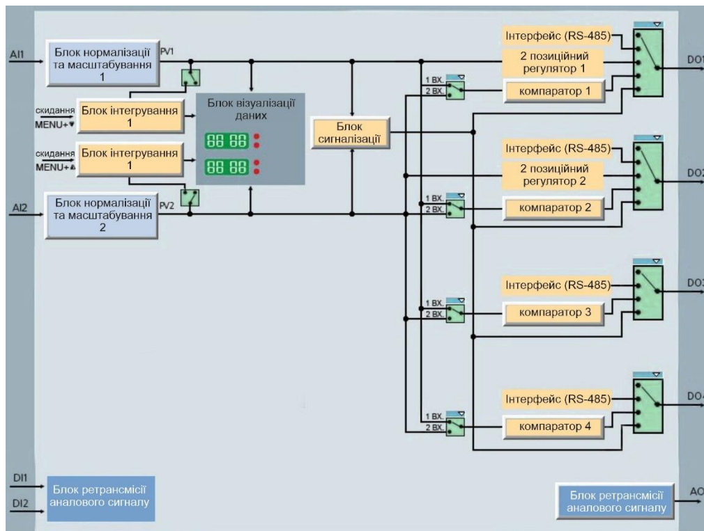
Рисунок 3.3 – Функціональна схема індикатора ІТМ-120-К6
