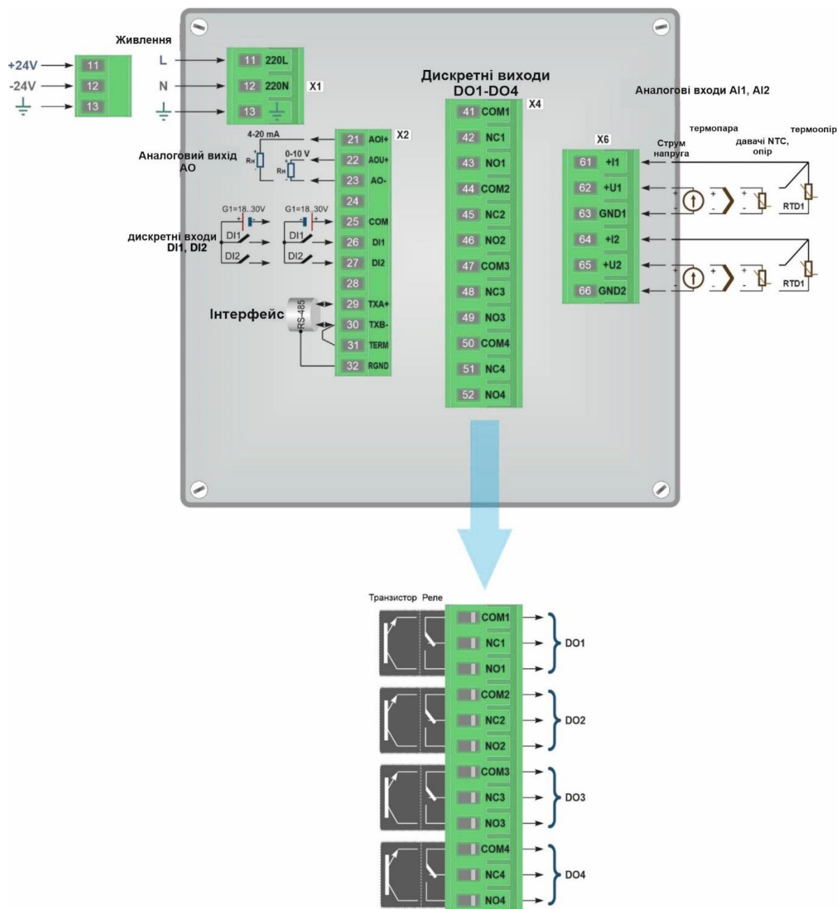
Рисунок Б.1 – Схема зовнішніх з'єднань індикатора ITM-120-K6
