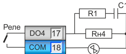
Рисунок Б.4 – Схема підключення індуктивного навантаження для механічного реле
