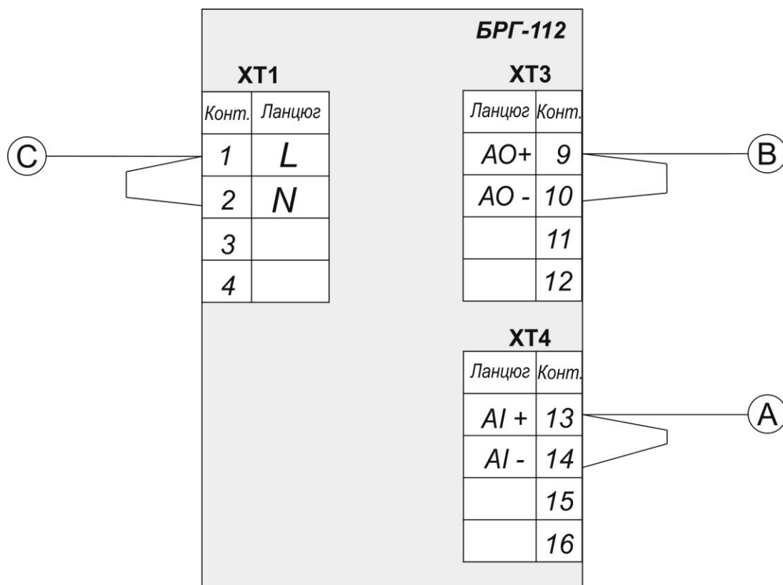
Рисунок Б.1 - Схема перевірки опору ізоляції
