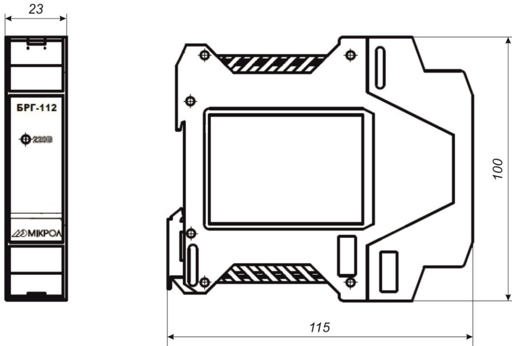
Рисунок 1.1 - Зовнішній вигляд і габаритні розміри блоку БРГ-112
