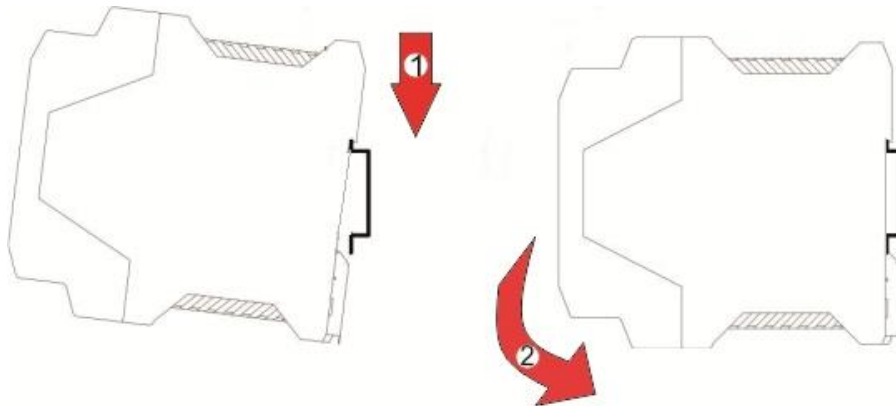
Рисунок 3.2 – Схема кріплення блоку БРГ-112 на DIN-рейку
