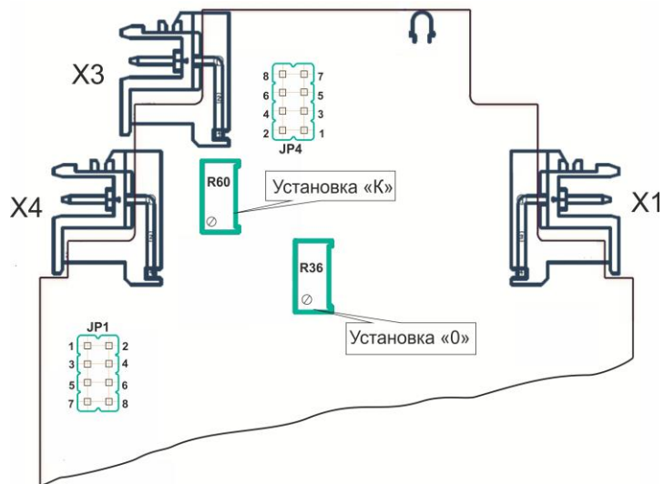
Рисунок 3.1- Розміщення блоків перемичок вибору вхідного і вихідного сигналів
