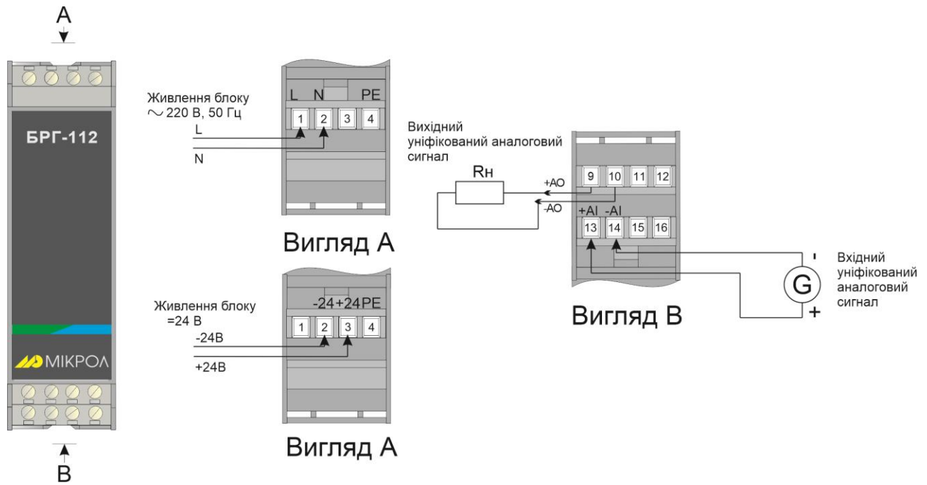
Рисунок 3.4 - Схема електричних підключень блоку БРГ-112
