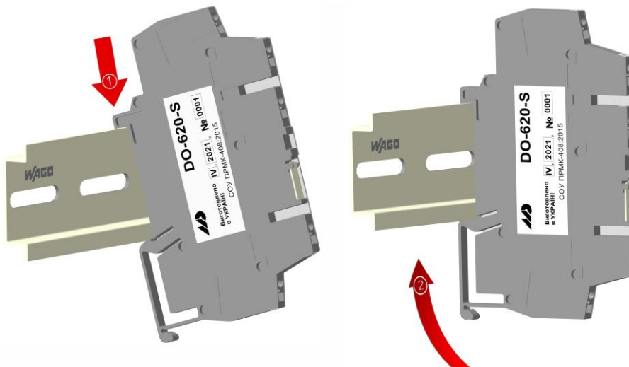
Рисунок 3.2 - Схема кріплення модуля DO-620-S на DIN-рейку
