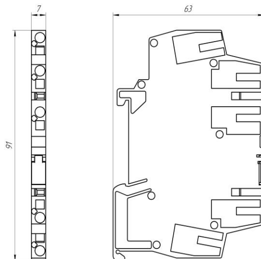
Рисунок 1.1 - Зовнішній вигляд і габаритні розміри модуля DO-620-S
