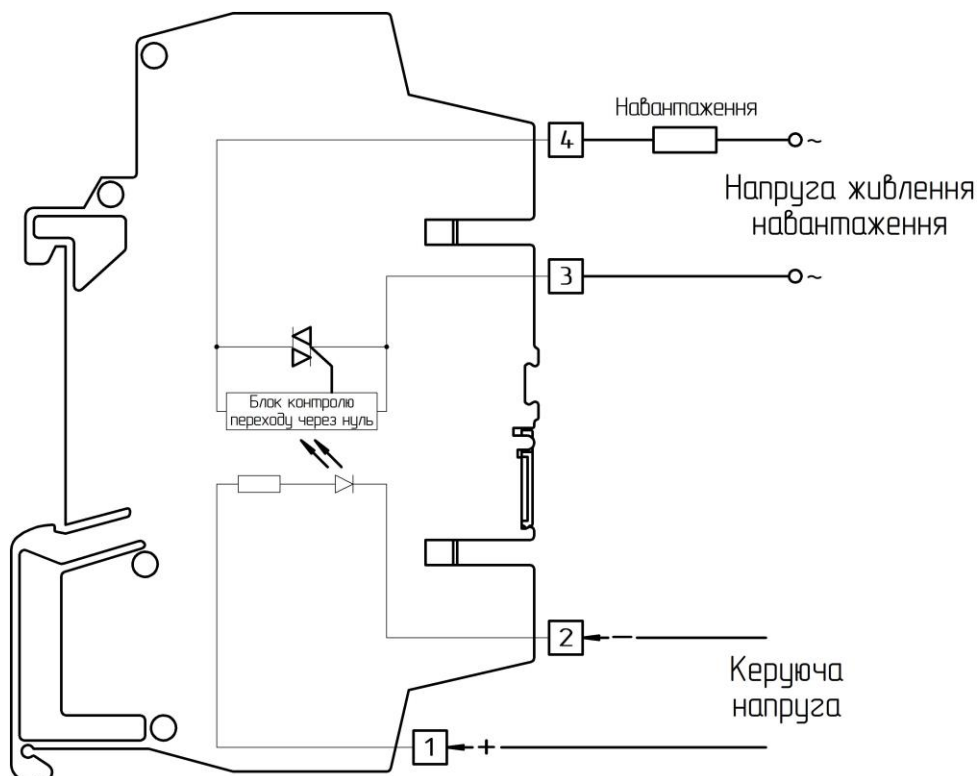
Рисунок 3.4 - Схема зовнішніх з'єднань модуля DO-620-S
