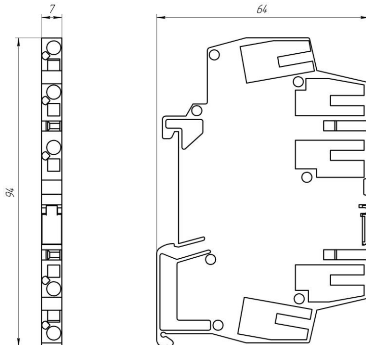
Рисунок 1.1 - Зовнішній вигляд і габаритні розміри перетворювача БПО-644
