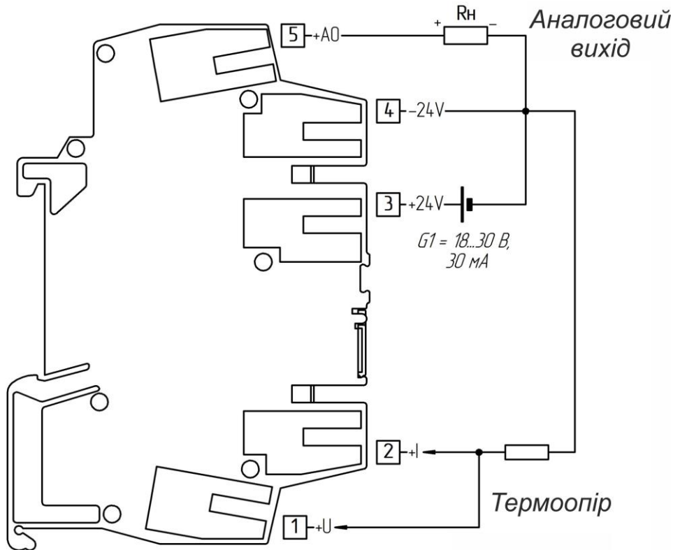
Рисунок 3.3 - Схема зовнішніх з'єднань перетворювача БПО-644
