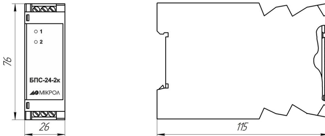
Рисунок 1.1 – Внешний вид и габаритные размеры БПС-24-2к-Н15
