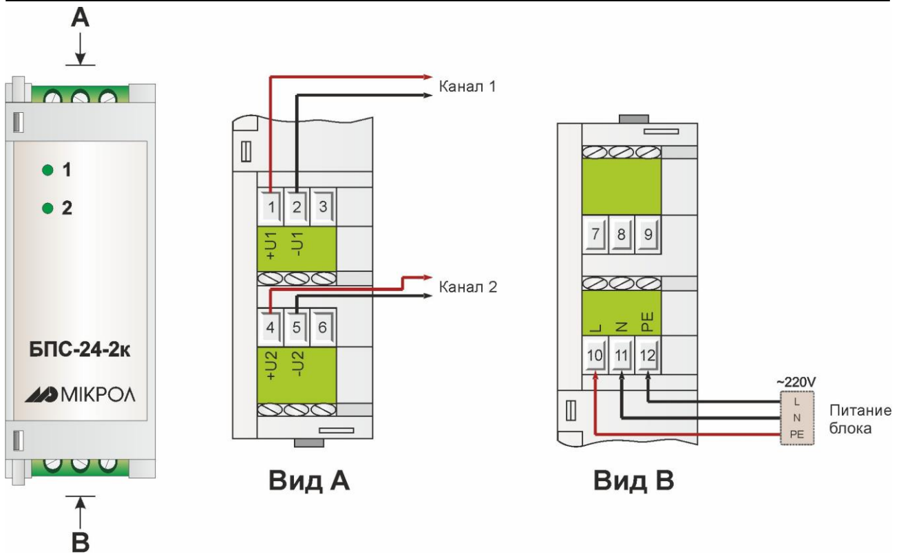
Рисунок 3.3 – Схема внешних соединений БПС-24-2к-Н15
