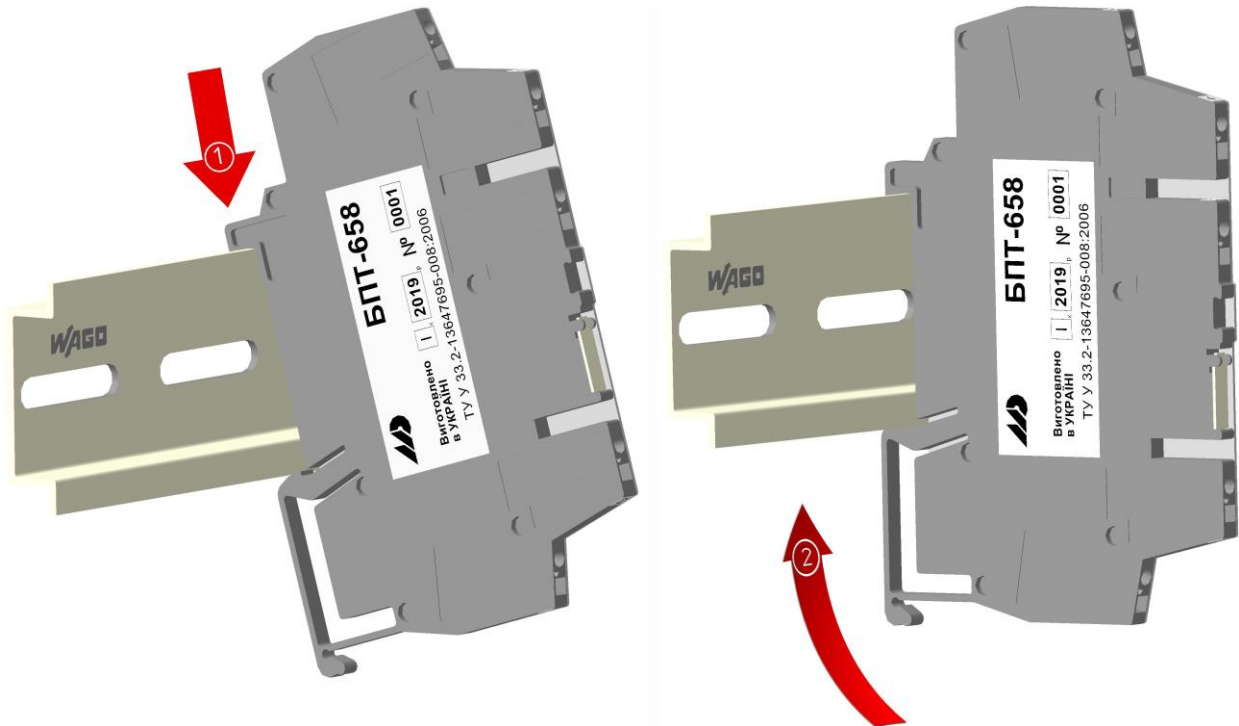
Рисунок 3.2 – Схема крепления преобразователя БПТ-658 на DIN-рейку
