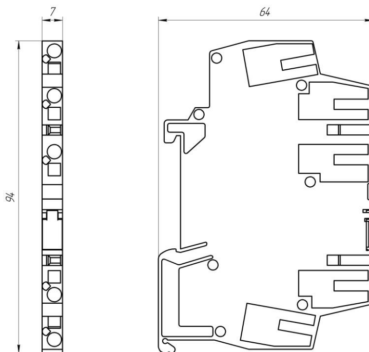
Рисунок 1.1 – Внешний вид и габаритные размеры преобразователя БПТ-658
