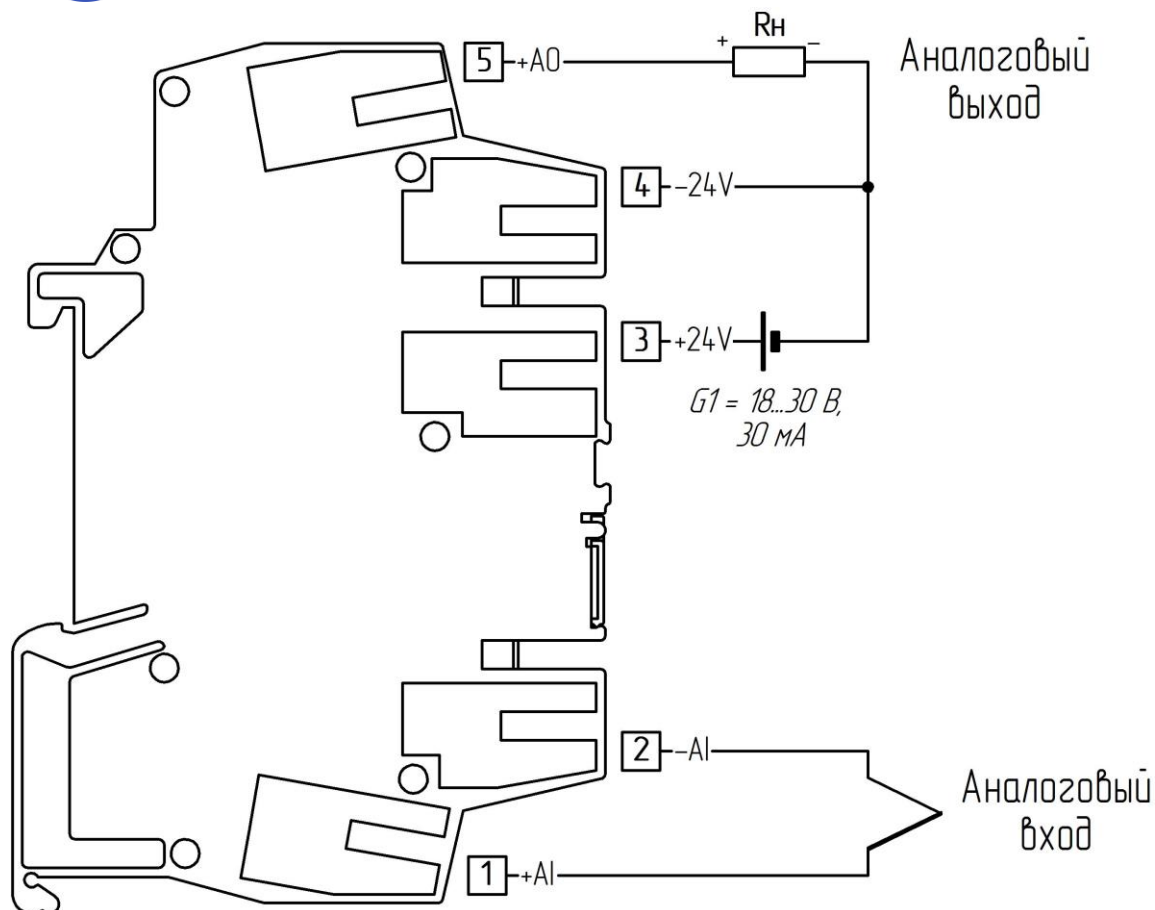
Рисунок 3.4 - Схема внешних соединений преобразователя БПТ-658
