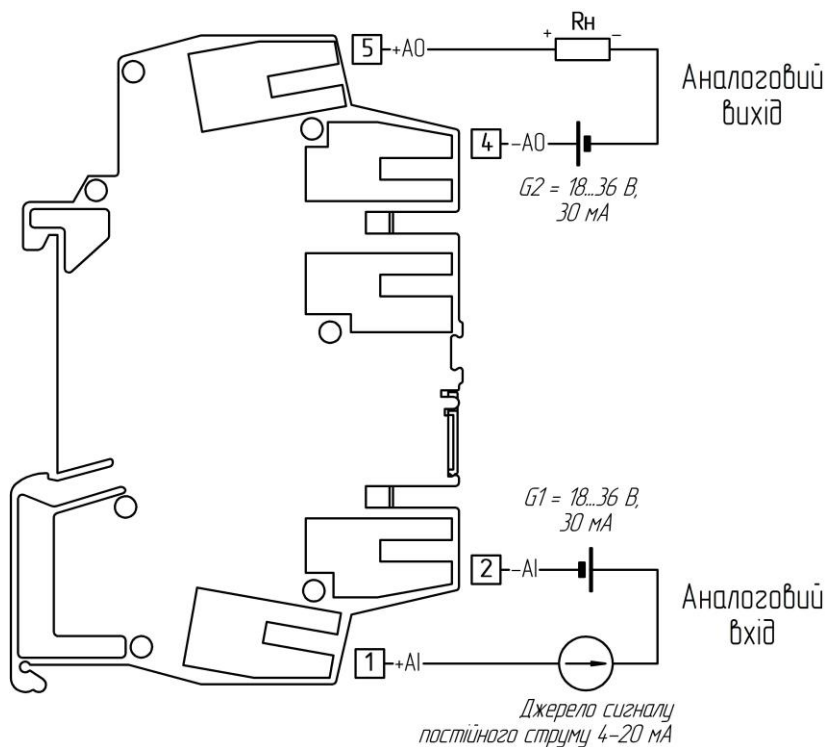
Рисунок 3.4 - Схема зовнішніх з'єднань блоку BPG-670
