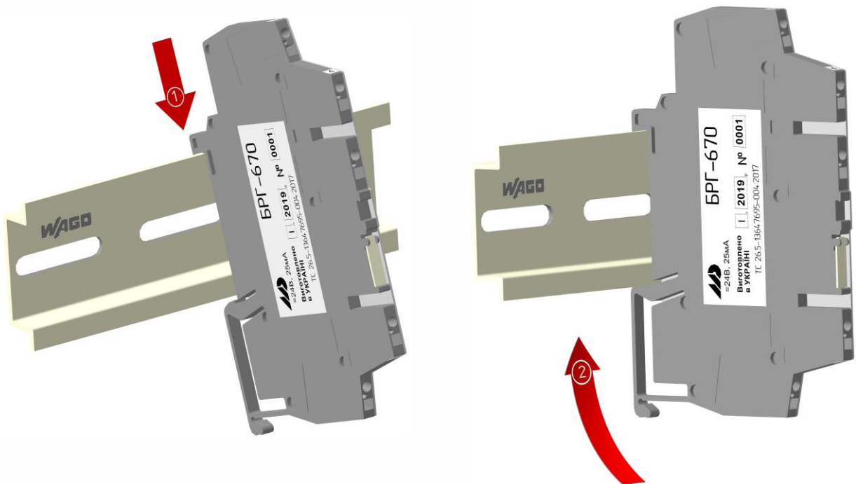
Рисунок 3.2 - Схема кріплення блоку BPG-670 на DIN-рейку
