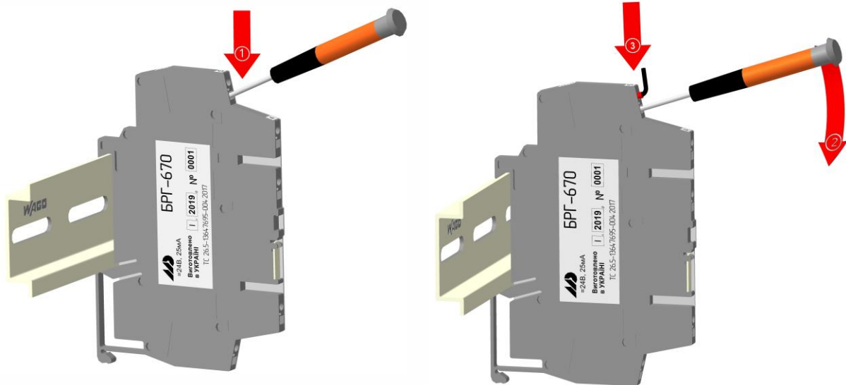
Рисунок 3.3 - Схема установки дротів за допомогою плоскої викрутки
