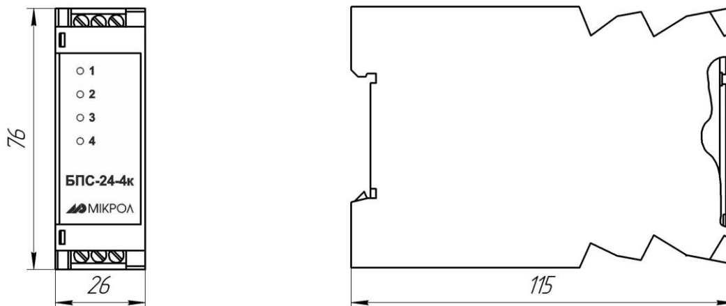
Рисунок 1.1 – Внешний вид и габаритные размеры БПС-24-4к-Н15
