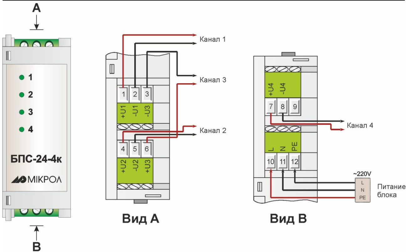
Рисунок 3.3 – Схема внешних соединений БПС-24-4к-Н15
