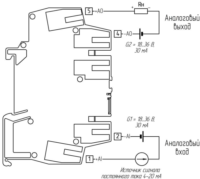
Рисунок 3.4 - Схема внешних соединений блока БРГ-670
