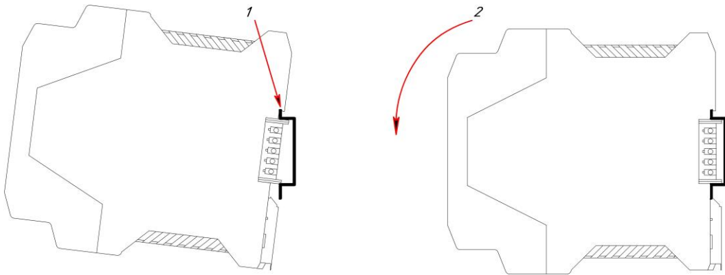
Рисунок 3.2 – Схема крепления преобразователя ПНС-102 на DIN-рельсе
