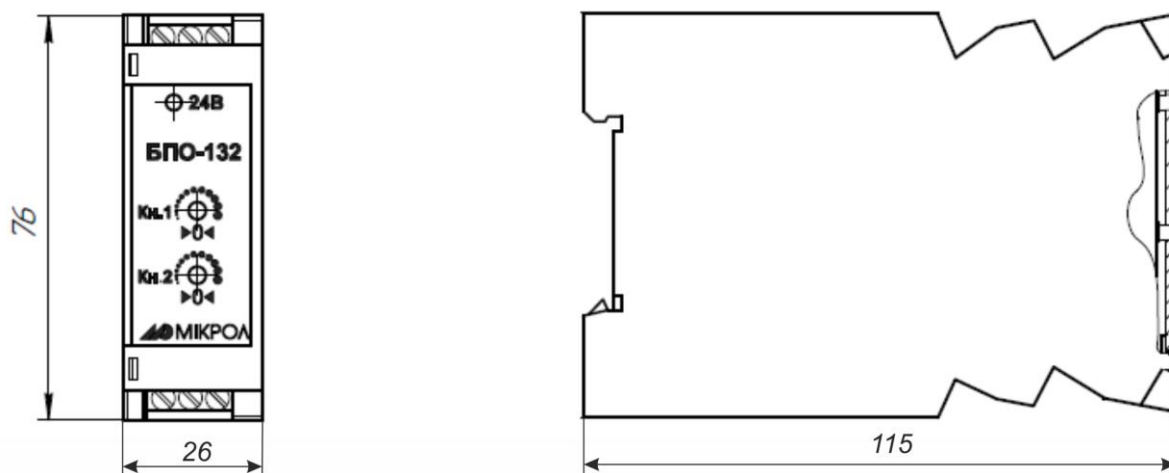
Рисунок 1.1 – Внешний вид и габаритные размеры БПО-132
