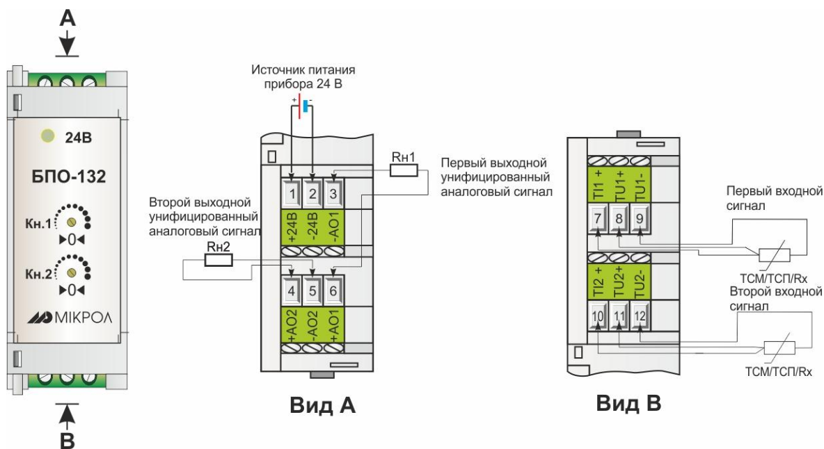
Рисунок 3.3 - Схема электрическая подключений блока БПО-132
